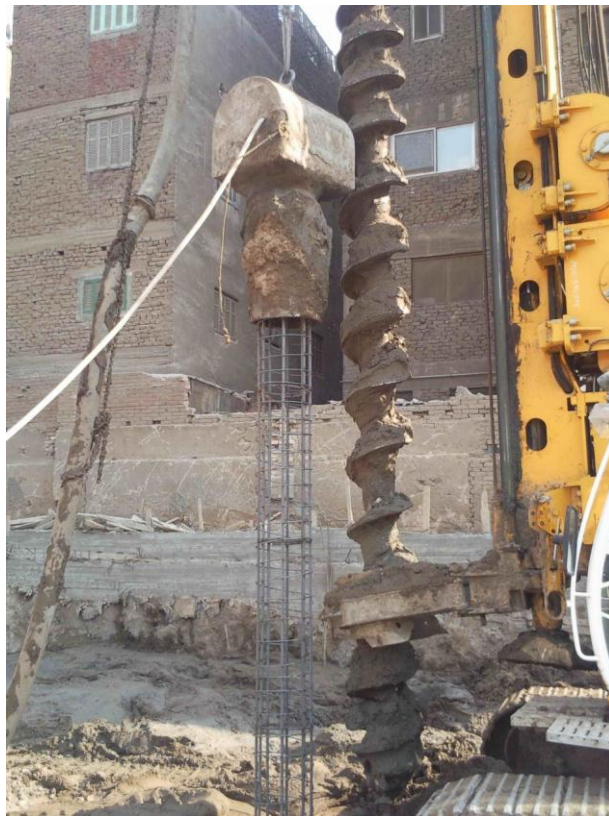
عملية إنزال التفقيصة بواسطة الهزاز
