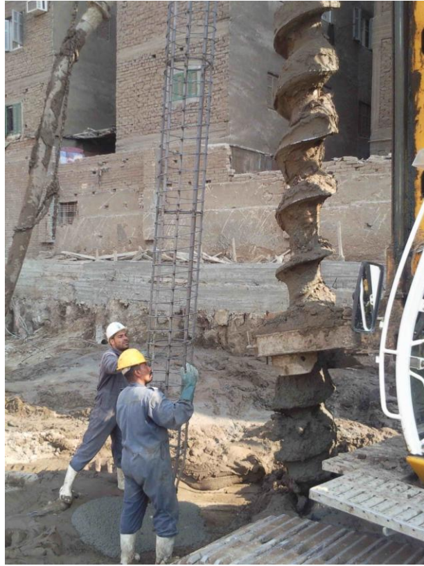
بدء إنزال التفقيصة الحديد بالخازوق
