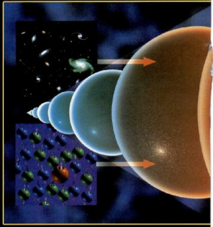
• الانفجار العظيم
