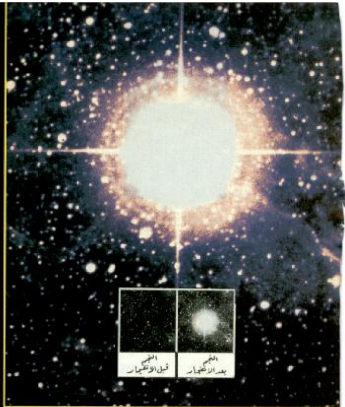
● انفجار نجم
