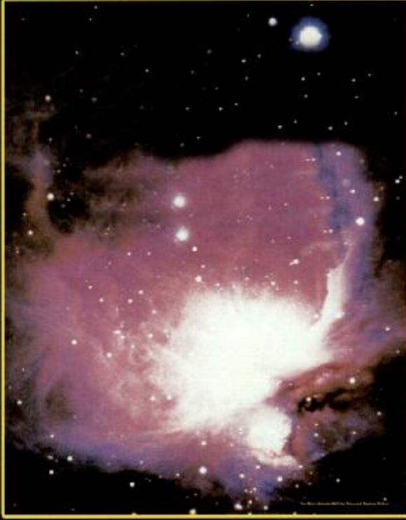
• اتساع الكون
