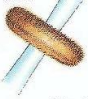
مجرة راديوية
