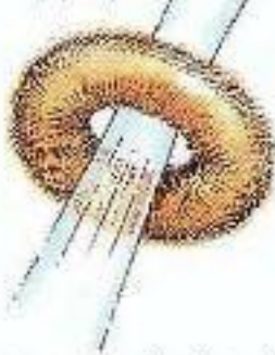
شبه نجم
