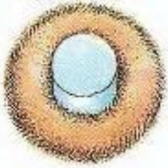
مجرة الشعلة
