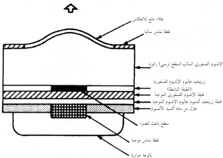
الشكل 4-7 بنية صمام زرنيخيد غاليوم الإنديوم الفسفوري / الإنديوم الفسفوري الثنائي باعث للضوء ذو الكفاءة الإشعاعية العالية.
