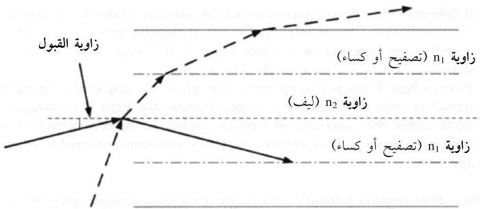
الشكل 2-12 زاوية القبول للضوء الساقط على واجهة نهائية لليف البصري.
