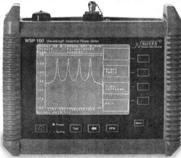
الشكل 8-13 عداد قدرة انتقاء متعدد الأطوال الموجية (WSP100) - (تقدمة شركة نويانس (Noynes).
