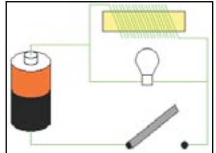
● شكل (١) جهاز الحث الكهربائي.
