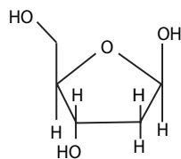
Deoxyribose
