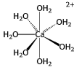
Calcium ion
