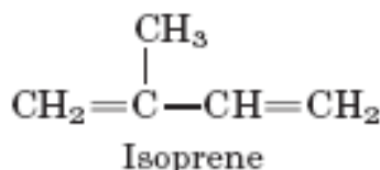
الشكل (7-23): الأيزوبرين.
