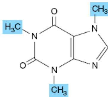
الشكل (6-8): الكافائين.
