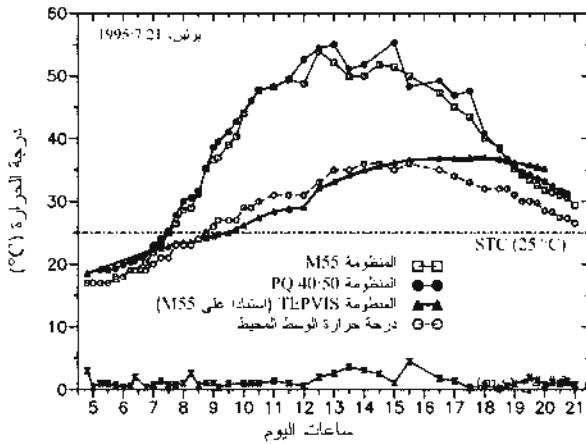
الشكل (10-18): درجات الحرارة للمنظومة TEPVIS مقارنة بمنظومتين فولتضوئيتين تقليديتين (MP55، PQ 10/40)، جميعها تم تشغيلها عند نقطة القدرة القصوى، مع درجة حرارة الوسط المحيط وسرعة الرياح ليوم صافى في برلين بألمانيا (7/21/1995).
