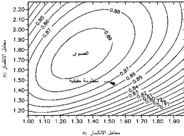
الشكل (10-6): النفاذية البصرية لتغليف منظومة كدالة في معامل الانكسار للوجين العفلاتيين العلويين (شريحتين بصريتين) للسقوط العمودي للإشعاعية (\theta = 0^\circ) .
