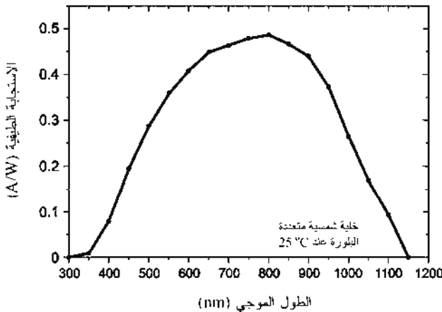
الشكل (2-5): الاستجابة الطيفية الفعلية لخلية شمسية سليكونية متعددة البلورة (نوع ASE).
