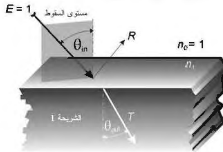
الشكل (14-7): النفاذية والانعكاسية عند الحد الفاصل للسقوط غير الرأسي للضوء ( \theta_{in} \neq 0^\circ ).
