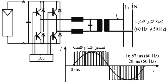
الشكل (3-3): مخطط لدائرة عاكس جيبى أحادي الطور يستند على تضمين اتساع النبضة لحقق الفولتضونية في الشبكة.
