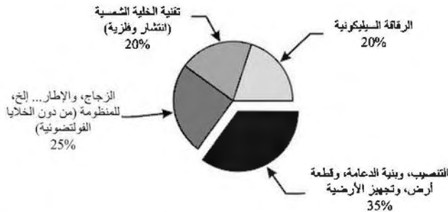
الشكل (2-17): توزيع التكاليف على تنصيب محطة قدرة فولتضوئية صغيرة (من دون تكيف القدرة الكهربائية) (Goetzberger) (1994).
