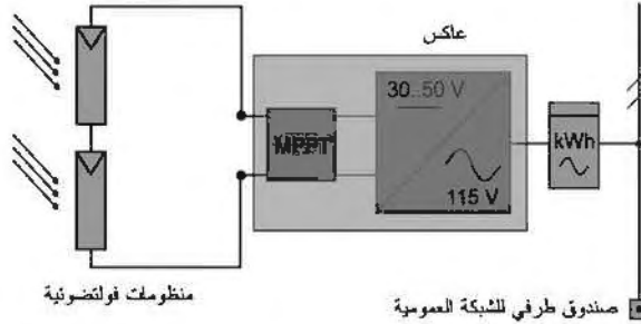
الشكل (2-3): مخطط لنظام حقن شبكي فولتضوئي نموذجي أحادي الطور مجهز بمتعقب لنقطة القدرة القصوى (Maximum-Power-Point Tracker (MPPT) وعداد الطاقة (kWh).
