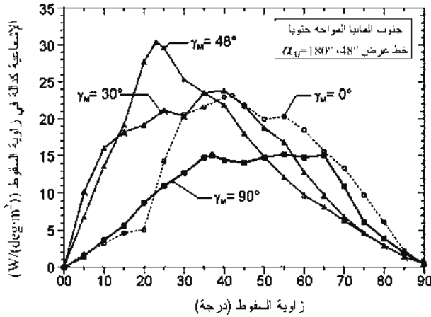
الشكل (7-10): الإشعاعية كدالة في زاوية السقوط لزاويا ارتفاع مختلفة \gamma_m للمنظومة الفولتضوئية في مدينة فريبيرج بألمانيا (48° N)، وفقاً لـ (Prev [et. al.] 1995).
