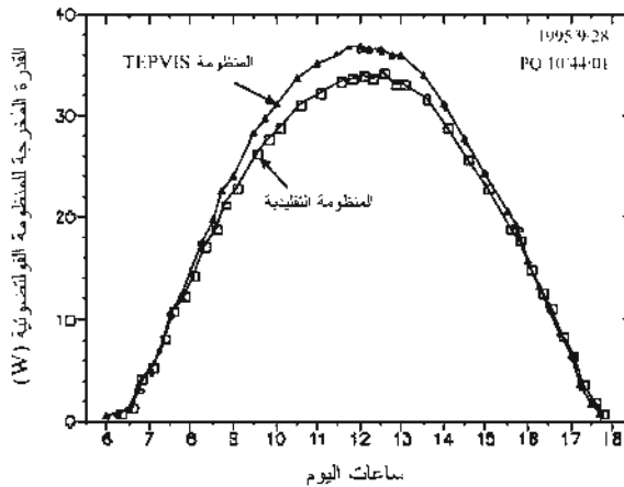
الشكل (10-24): القدرة الكهربائية المُخرَجة عند نقطة القدرة القصوى للمنظومة TEPVIS خلال يوم صافى مقارنة بمنظومة فولتضوئية تقليدية (بولايو، زيمبابوي، 38^{\circ}37' E, 20^{\circ}10' S ).
