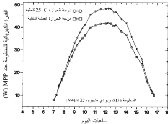
الشكل (10-16): القدرة الكهربائية المُخرَجة المقاسة لظروف حقيقية مقارنة بالقدرة المُخرَجة النظرية عند درجة حرارة ثابتة 25^{\circ}\text{C} للخلية (ظروف نقطة القدرة القصوى (MPP) لكلتا المنحنيين).
