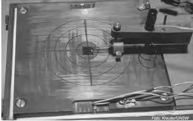
الشكل (2-6): جهاز لقياس خصائص التيار-الجهد ( I-V )، والكفاءة، والاستجابة الطيفية. واتشكل مبنين مع خلية شمسية ذات كفاءة عالية في جامعة نيو ساوث ويلز (UNSW).
