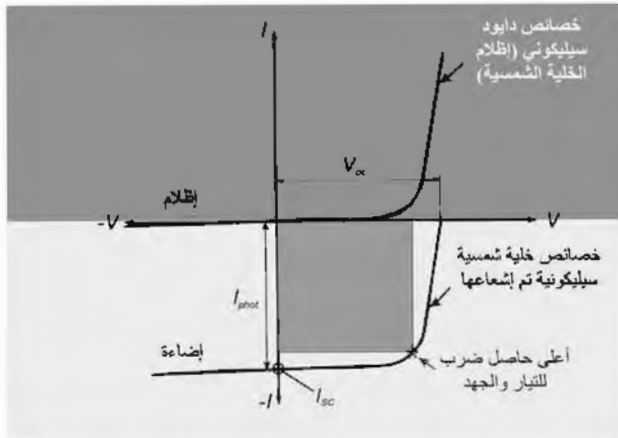
الشكل (2-3): خصائص التيار-الجهد لداوود (إظلام الخلية الشمسية) و خلية شمسية تم إشعاعها مع تيار دائرة القصر I_{sc} وجهد الدائرة المفتوحة V_{oc} .
