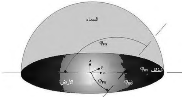
الشكل (7-22): تعريف عوامل الرؤية \phi لتبادل الإشعاع الحراري بين المنظومة الشمسية الأرضية، والسماء، والأرض.
