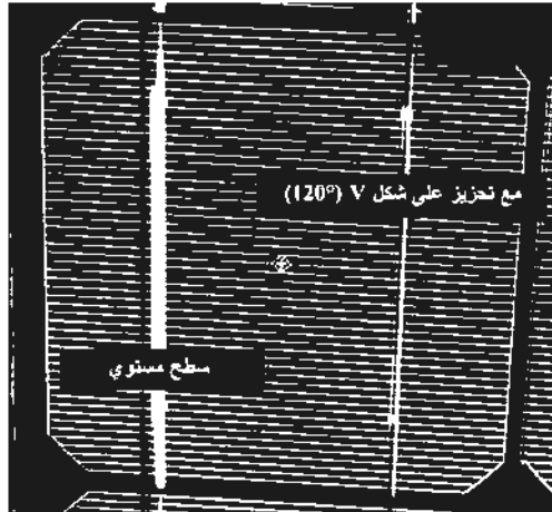
الشكل (10-3): الأيسر: سطح منظومة عادي مستوي. الأيمن: انخفاض بصري لعرض شريط التلامس (القضيب الموصل) بتطبيق جز على شكل V على السطح الواقع أعلى التلامس.
