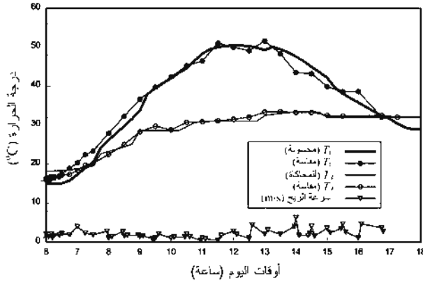
الشكل (7-25): مقارنة درجة الحرارة المحاكاة للخلية الشمسية بدرجة الحرارة الفعلية المقاسة خلال اليوم (منطقة فولدرز غاب في أستراليا، 21 آذار/ مارس 1994، سماء صافية).
