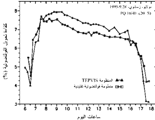
الشكل (10-23): مقارنة كفاءة تحويل الفولتضوئية لمنظومة فولتضوئية تقليدية متعددة البلورة بالمنظومة TEPVIS خلال يوم صافى في بولايو بزمبابوي.
