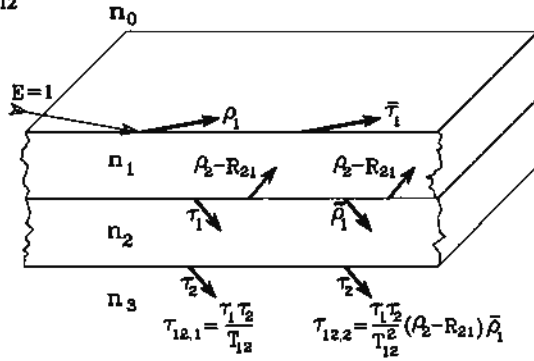
الشكل (7-16): النفاذية لنظام بصري يتكون من شريحتين بصريتين.
