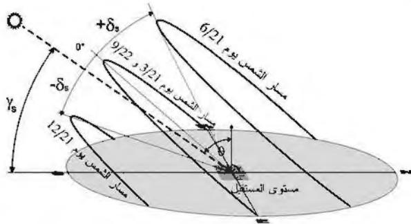
الشكل (3-7): مسار الشمس على نصف الكرة الشمالي في الاعتدالين الخريفي والربيعي (9/22 و 3/21)، والصيف (6/21)، والشتاء (12/21)، ومبين أيضاً الانحرافات القوسية \delta_s لنقاط منتصف اليوم وزاوية الارتفاع الفعلية للشمس \gamma_s مع زاوية السقوط \theta_m على مستوى المسطح (Ertürk 1997).
