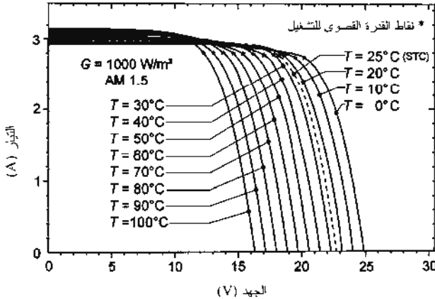
الشكل (2-11): خصائص التيار الجهد لمنظومة فولتضوئية سليكونية متعددة البلورة عند درجات حرارة مختلفة (مع ثبات الإشعاعية والطيف عند 1,000 \text{ W/m}^2 و AM 1.5).
