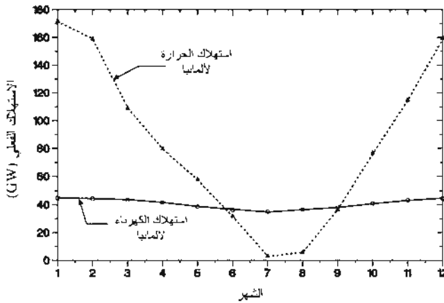
الشكل (1-أ): منحني استهلاك القدرة الموسمي لغرب ألمانيا: أحمال الكهرباء والحرارة خلال سنة نموذجية (المراجع: هينلوث (Heinloth) 1996).
