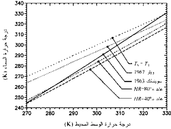
الشكل (23-7): درجة حرارة السماء T_s كدالة في درجة حرارة الوسط المحيط T_a محسوبة باستخدام نماذج مختلفة.
