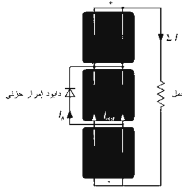
الشكل (2-13): رسم تخطيطي يوضح تشغيل دايود الإمرار الجزئي: خلية شمسية مع تظليل جزئي في سلسلة مكونة من 3 خلايا متصلة على التوالي.
