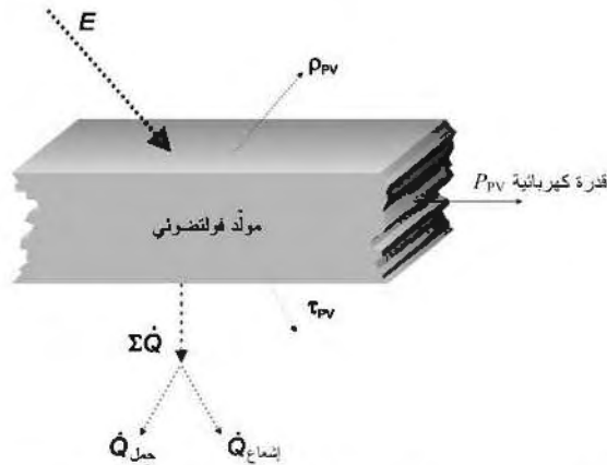
الشكل (7-20): رسم تخطيطي لتدفقات الطاقة الداخلة والخارجة لمنظومة فولتضوئية (تدفقات الطاقة البصرية رسمت كخطوط منقطعة، والحرارية كخطوط منقطعة، والكهربائية كخطوط كاملة، وسماعة الخط يمثل القيمة النموذجية للتدفقات).
