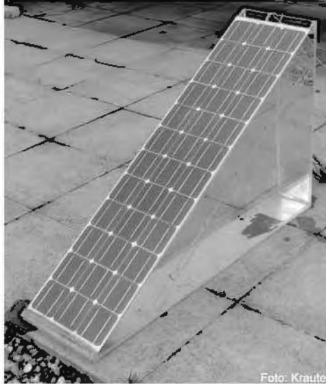
الشكل (10-17): منظومة فولتضوئية محسنة حرارياً بحامل مدمج (TEPVIS): نموذج إثبات الفكرة مصنوعة من الأكرليك أظهر كسباً 11.6% في المردود الكهربائي (برلين، ألمانيا، 1995).
