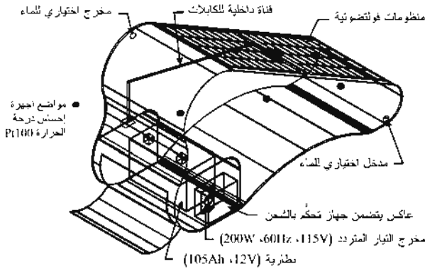
الشكل (10-25): التركيب الداخلي للنظام المنزلي الشمسي المتكامل (I-SHS).
