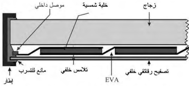
الشكل (8-2): مقطع عرضي لخلاية فولتضوئية مصفحة.
