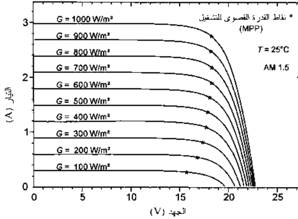
الشكل (2-10): خصائص التيار-الجهد لمنظومة فولتضوية سليكونية متعددة البلورة لقيم إشعاعية مختلفة (مع شات درجة الحرارة والمليف عند 25 °C و AM 1.5).
