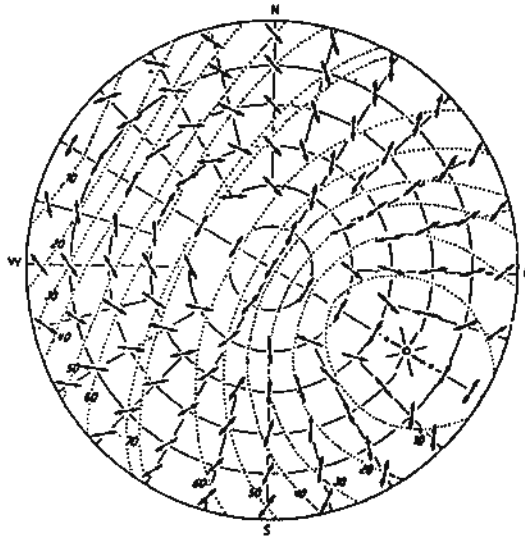
الشكل (7-11): نموذج استقطاب لنصف الكرة السماوي ليوم صاف ولزاوية ارتفاع للشمس 30° (فون فريش (von Frisch)، 1965).
