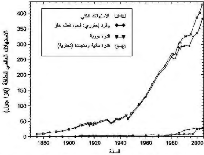
الشكل (1-1): الاستهلاك العالمي للطاقة الأساسية بالإكزا جول (EJ) ( 10^{18} جول) كدالة في الزمن لأعوام (1875 - 2004) مع إسهامات الوقود الباعثة والخالية من ثاني أكسيد الكربون المصادر: 1875-1965: Interatom-Shell-Study 1992, 1970-1988: UN yearbook of World Energy Statistics, 1989 - 2004: BP Statixtic Review of World Energy, 1996.
