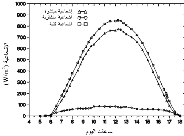
الشكل (10-14): الإشعاعية الأفقية الكلية، والمباشرة، والانتشارية في الاعتدال (1994/9/22) في مدينة ريو دي جانيرو بالبرازيل (22°54' S, 43°13' W).
