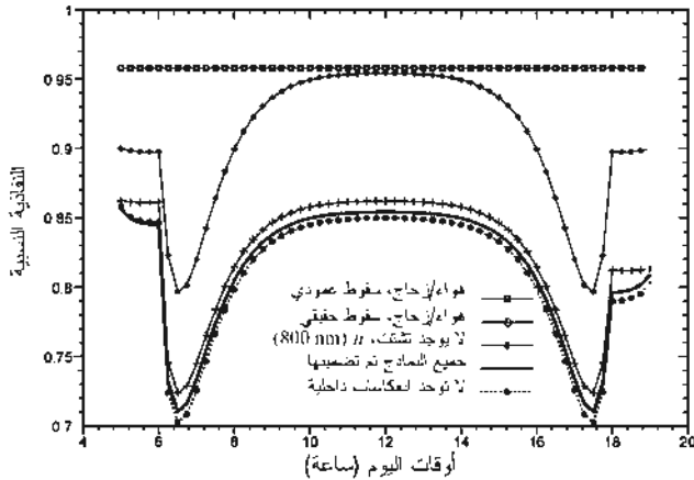
الشكل (7-19): النفاذية خلال منظومة فولتضونية ليوم صاف باستخدام نماذج مختلفة (من دون امتصاص)
