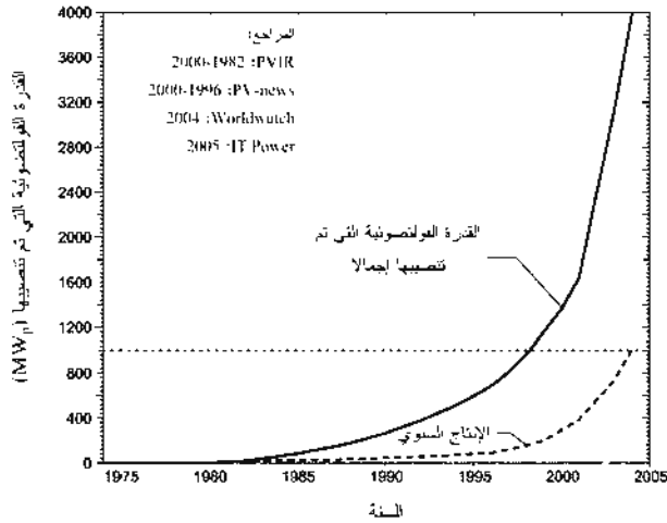
الشكل (21-2): تطور حرق الفولتضوئية؛ السعة التي تم تنصيبها والإنتاج السنوي (المراجع: احبار الفولتضوئية (PV-news) وتقرير اساطعين على الفولتضوئية (PVIR) Photovoltaic Insiders Report - 2000-1982، ومعهد المراقبة العالمية (Worldwatch Institute) - 2004، وتقنية معلومات القدرة (IT Power) - 2005).
