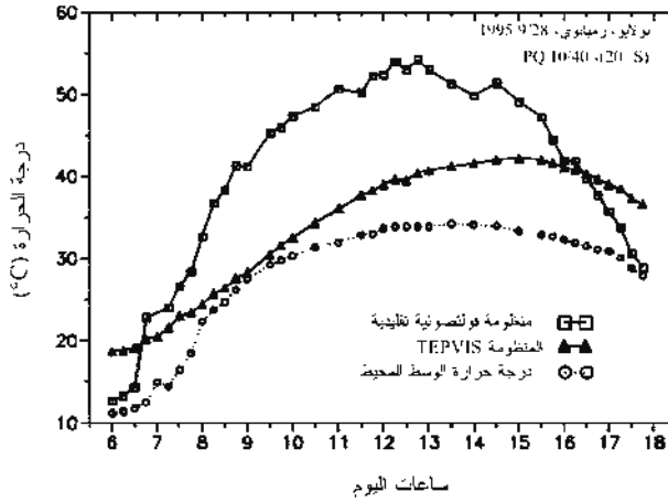
الشكل (10-22): مقارنة درجات الحرارة لمنظومة فولتضوئية تقليدية متعددة البلورة بالمنظومة TEPVIS (كلاهما استناداً إلى المنظومة PQ 10/40) خلال يوم صافٍ في بولايو بزيمبابوي (38°37' E, 20°10' S).
