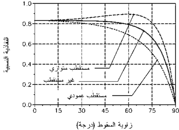
الشكل (7-18): النفاذية لنظام بصري يتكون من ثلاث شرائح كدالة لزاوية السقوط.
