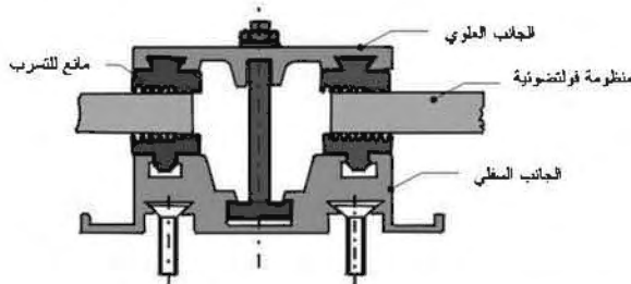
الشكل (2-15): مقطع عرضي لمركّب التثبيت للمنظومات الفولتضوئية اللاإطارية (شميد (Schmid) 1988).
