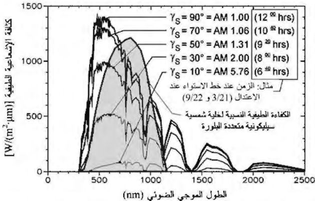
الشكل (2-7): الاستجابة الطيفية الفعلية لخلية شمسية متعددة البلورة (نوع ASE) مع الطيف الشمسي لزاويا ارتفاع مختلفة للشمس، والكتل الهوائية المكافئة (AM)، والزمن عند خط الاستواء للاعتدال.
