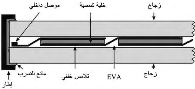
الشكل (9-2): مقطع عرضي لخلاية فولتضوئية مغلقة.
