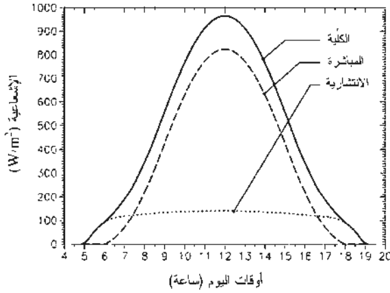
الشكل (5-7): الجزآن المباشر والانتشاري للإشعاعية الكلية ليوم صاف 3/21 (و 9/22) لمستقبل له زاوية الارتفاع نفسها كما لحظ العرض (36°)، وبالتالي تسقط أشعة الشمس عمودياً عند الظهيرة.
