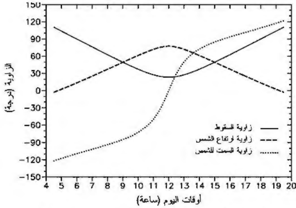
الشكل (2-7): زاوية ارتفاع الشمس \gamma_s ، وزاوية سمت الشمس \alpha_s ، وزاوية السقوط \theta_m على سطح المنظومة خلال يوم صيفي (21 يونيو)، خط عرض 36^\circ N، وزاوية ارتفاع المنظومة \gamma_M = 36^\circ موجهة نحو الجنوب).
