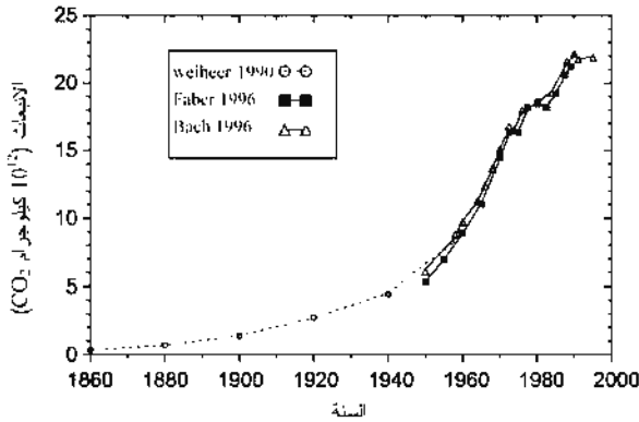
الشكل (1-3): الانبعاثات العالمية البشرية المنشأ لثاني أكسيد الكربون خلال الأعوام (1860-1995) وفقاً لويهير (Weiheer) 1990، وفابر (Faber) 1996، وباخ (Bach) 1996، والرصد العالمي (Worldwatch) 2000.
