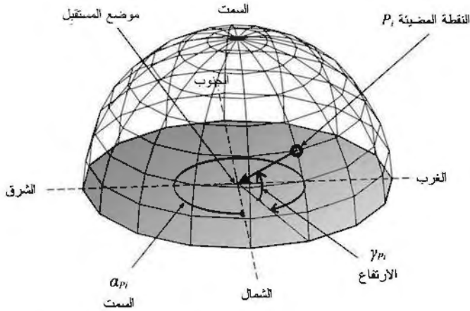
الشكل (1-7): تعريف زاوية الارتفاع \gamma_s وزاوية السمت \alpha_s لنقطة مضئبة P_i (الشمس، مثلاً) طبقاً للنموذج DIN 5034 الجزء 2.
