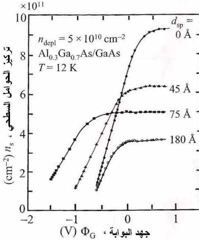
الشكل 7.7: علاقة كثافة القناة لإلكترونات ثنائية البعد بجهد البوابة المقيس في بني \text{Al}_{0.3}\text{Ga}_{0.7}\text{As}|\text{GaAs} عند T=12\text{ K} . ومن أجل سماكات فاصل مختلفة d_{sp} . كل العينات من السيليكون المشاب N_D = 4.6 \times 10^{17} \text{ cm}^{-3} ما عدا حالة السماكة 180 \text{ \AA} التي تكون فيها قيمة التركيز N_D = 9.2 \times 10^{17} \text{ cm}^{-3} وتكون سماكة طبقة \text{Al}_{0.3}\text{Ga}_{0.7}\text{As} المشابة مساوية 700 \text{ \AA} 1200
