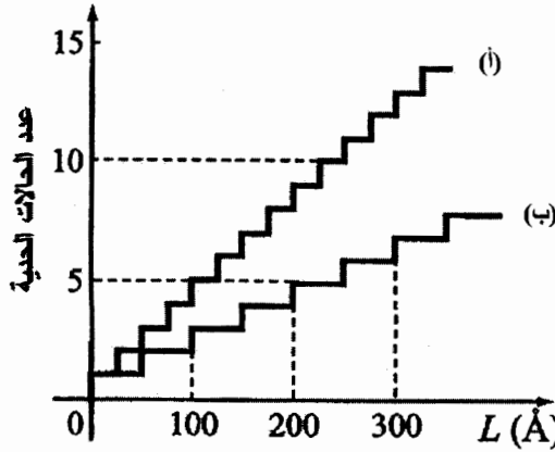
الشكل 5.3: عدد الحالات الحدية لبئر مربع بدلالة سماكة البئر: (أ) V_b=224\text{meV} ؛ m=0.4 m_0 ؛ (ب) V_b=150\text{meV} ؛ m=0.067m_0
