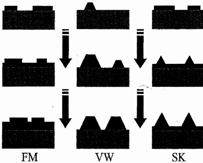
الشكل 16.5: أنماط النمو الطبقي الهجين الثلاثة: فرانك- فان ديرمير (FM)، فولمير وبيير (VW)، وسترانسكي كراستاتوف (SK)
