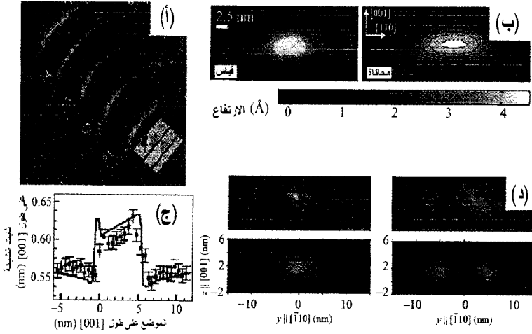
الشكل 9.5: مجهر المسح النفقي المقطعي: (أ) صورة ركام من جزر InAs في GaAs؛ (ب) مقارنة بين خطوط التسوية المقيسة والمحاكاة من أجل عينة مشابهة؛ (ج) معامل الشبكة في اتجاه النمو في جزيرة InAs (حصلنا على المعطيات التجريبية بمجهر مسح نفقي مقطعي). الخط المستمر ناتج عن محاكاة فرص تزايد In من قاعدة الجزيرة إلى قمته L، (د) تابع الموجة الإلكتروني المقيس في حالة انحيازين مختلفين للطرف مقارنةً بالمحاكاة من أجل حالة الأرض وحالة الإثارة الأولى
