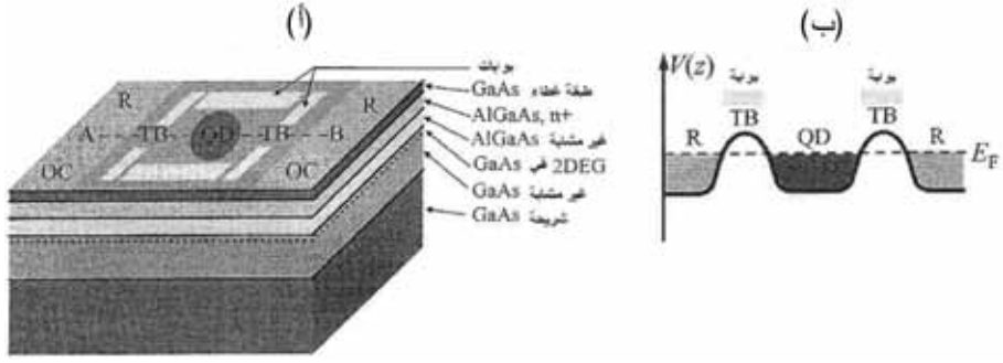
الشكل 23.8 (أ) نمذجة تصميم غاز ثنائي البعد على الهيئة المطلوبة من أجل التطبيقات الأحادية الإلكترون: التماس الأومي OC، خزان الإلكترونات R، النقطة الكمومية QD، الحاجز النفقي TB. (ب) منحنى الكمون V(z) على طول الخط A-B. لا تظهر التماسات الأومية OC لأنها خارج المنطقة الممثلة
