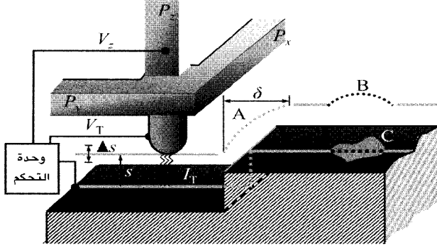
الشكل 8.5 مبدأ عمل المجهر النفقي الماسح
