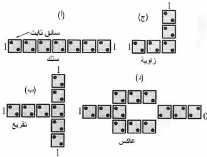
الشكل 69.8: أمثلة على مصفوفات مؤتمتات بالنقاط الكمومية الخليوية الأبسط: سلك أو زاوية أو تفريع وعاكس
