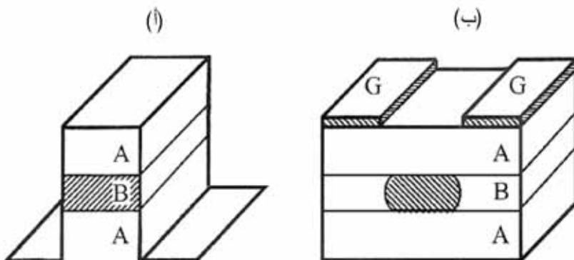
الشكل 9.7: تشكل السلك الكمومي بالحفر (أ) والبوباب المشطورة (ب) لغاز الإلكترونات الثنائي البعد.
