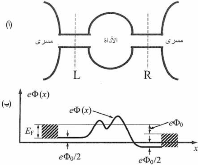
الشكل 17.6: (أ) مخطط بنية أداة ذات بنية نانوية ميزوسكوبية. (ب) منحني طاقة الكمون e \cdot \Phi(n) في الأداة الميزوسكوبية المستقطبة
