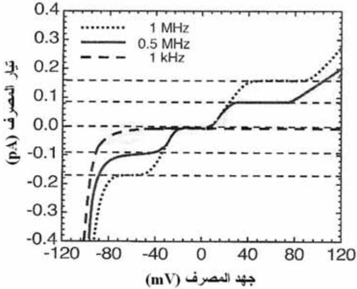
الشكل 29.8: تيار المصرف بدلالة جهد المصرف لأداة باب دوار. بيكو أمبير 10^{-12} \text{ PA} = \text{A}
