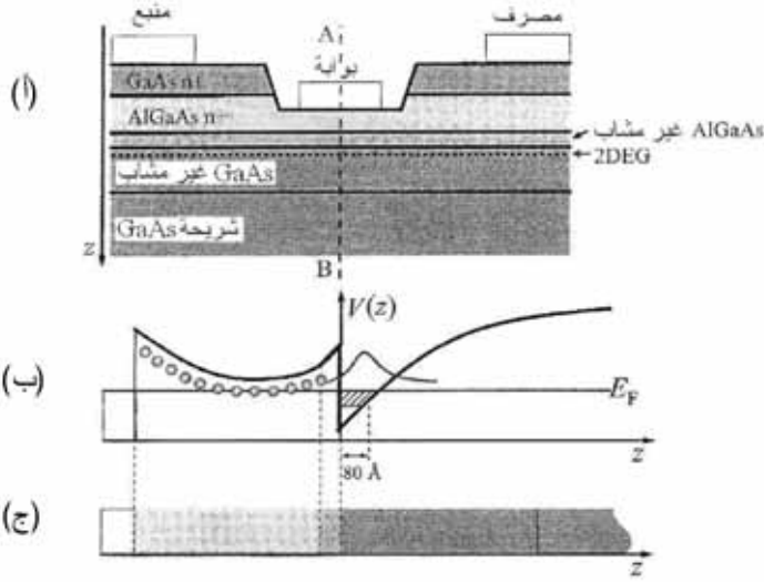
الشكل 13.8: ترانزستور البوابة المنكمشة n\text{-AlGaAs/GaAsFET} : (أ) مقطع HFETs (ب) مخطط حزم الطاقة على طول الخط A-B يظهر مستوى فيرمي وحالات حبس الإلكترونات في الطبقة المعطية هناك منطقتا نضوب لحاجز سميك: الأولى بسبب جهد شوتكي المتضمن، والثانية بسبب انزياح حزمة النقل عند الوصلة. (ج) سلسلة الطبقات على طول الخط A-B
