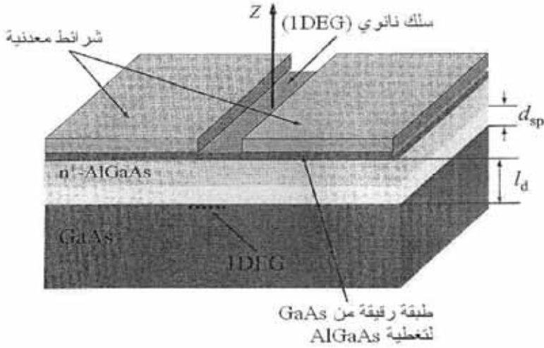
الشكل 22.8: سلك كمومي عند تواجده بنية متباينة GaAs/AIGaAs بمنطقتي نضوب تحت قطعتين معدنيتين منحازتين سلباً
