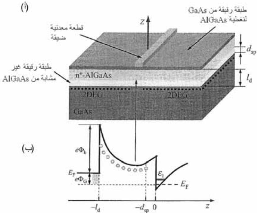
الشكل 21.8 (أ) غاز إلكتروني ثنائي البعد (2DEG، ممثلة بالخطوط المنقطعة) عند التواجه بين البنية المتباينة GaAs/AlGaAs المعدلة الإشابة مع طبقة نضوب تحت شريطة قطعة معدنية ضيقة (بوابة) منحازة سلباً. (ب) مخطط الحزم للبنية المتباينة GaAs/AlGaAs في منطقة البوابة. يدل الخط \epsilon_1 على الحزمة الجزئية الأدنى. يرمز \Phi_b إلى جهد شوتكي و \Phi_c إلى جهد البوابة
