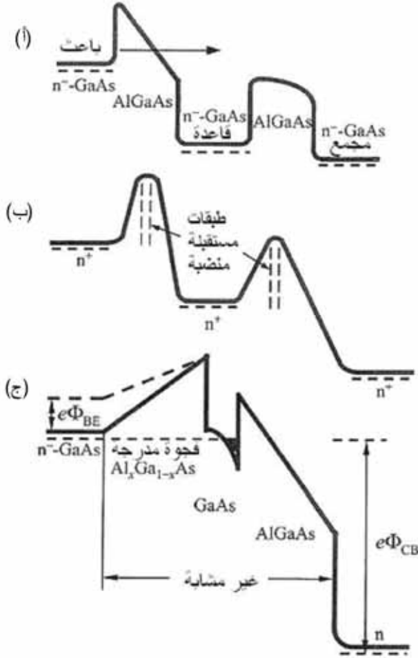
الشكل 38.8: مخططات حزم الطاقة من أجل الترانزستورات المقذوفية النصف الناقلة. (أ) بنية \text{AlGaAs/GaAs} مع أربع وصلات متباينة وقاعدة مشوبة. تحقن الإلكترونات في القاعدة بفضل العبور النفقي. ندعو هذا النوع من الأدوات مضخم النقل النفقي للإلكترونات الحارة. (ب) أداة إلكترون متباينة البنية. تتشكل الحواجز بإشابة p -مستوية. وتكون القاعدة مشابهة- n . (ج) أداة مع قاعدة غير مشابهة
