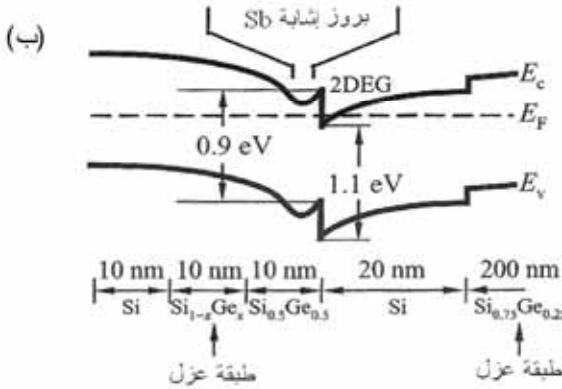
الشكل 14.8: الترانزستور MODFET بقناة n- وقاعدة Si/SiGe (أ) مقطع في الأداة: تتشكل قناة الإلكترونات في الطبقة المشدودة. (ب) مخطط حزم الطاقة للأداة
