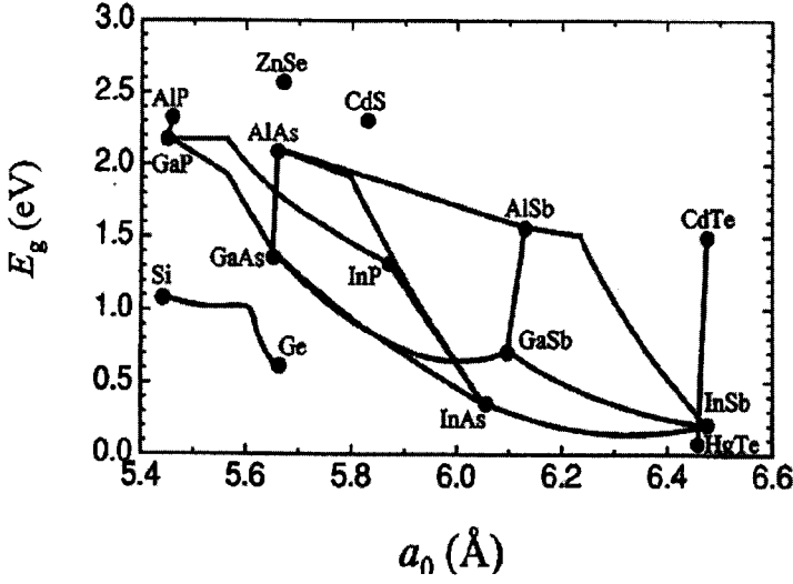
الشكل 14.4: فجوات حزم الطاقة بدرجة حرارة الغرفة E_g كتابع لثابت الشبكة a_0 من أجل مجموعة مركبات مختارة III-V و II-VI ومواد مختارة من المجموعة IV وخليطها
