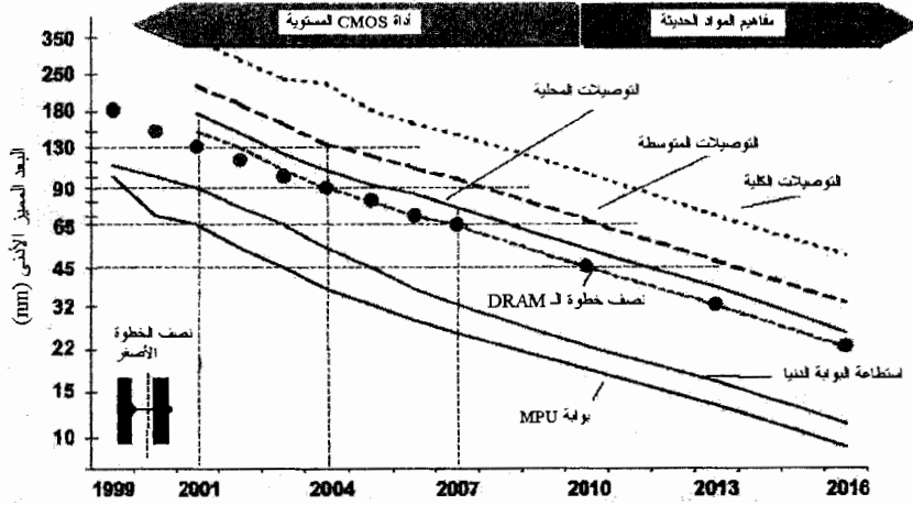
الشكل 1.1: عقد التفتحات وأبعاد بوابة الترانزستور الصغرى بتطبيق خارطة الطريق ITRS
