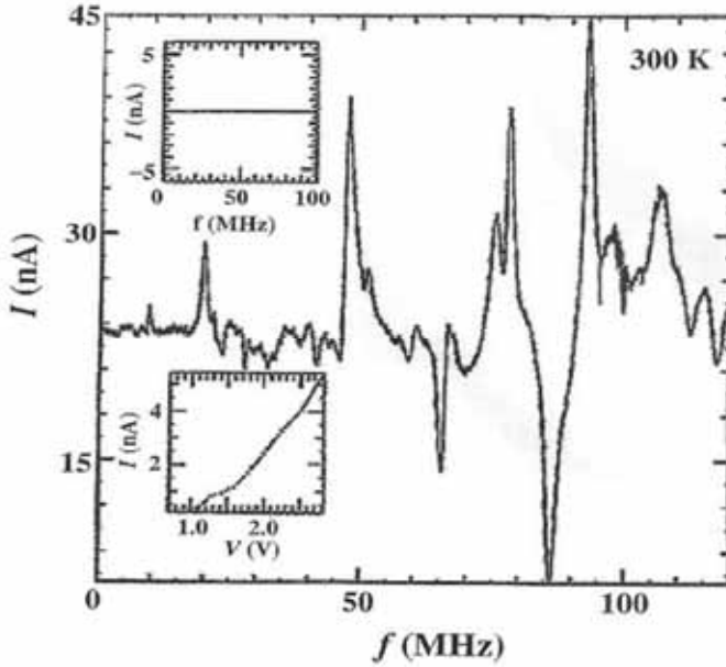
الشكل 64.8: التيار الكهربائي في المكوك الإلكتروني بدلالة التردد في دارة البوابة. النافذة العليا: الدعامة محجوزة ولا يوجد أي تيار. النافذة الدنيا: تيار المكوك כתابع لجهد المنبع - المصرف عند تردد معطى في دارة البوابة
