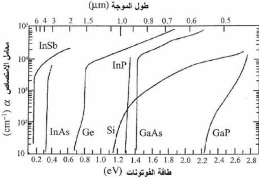
الشكل 42.8: معامل الامتصاص بدلالة طاقة الفوتون وطول الموجة من أجل الانتقالات الضوئية بين الحزم في أنصاف نواقل مختلفة
