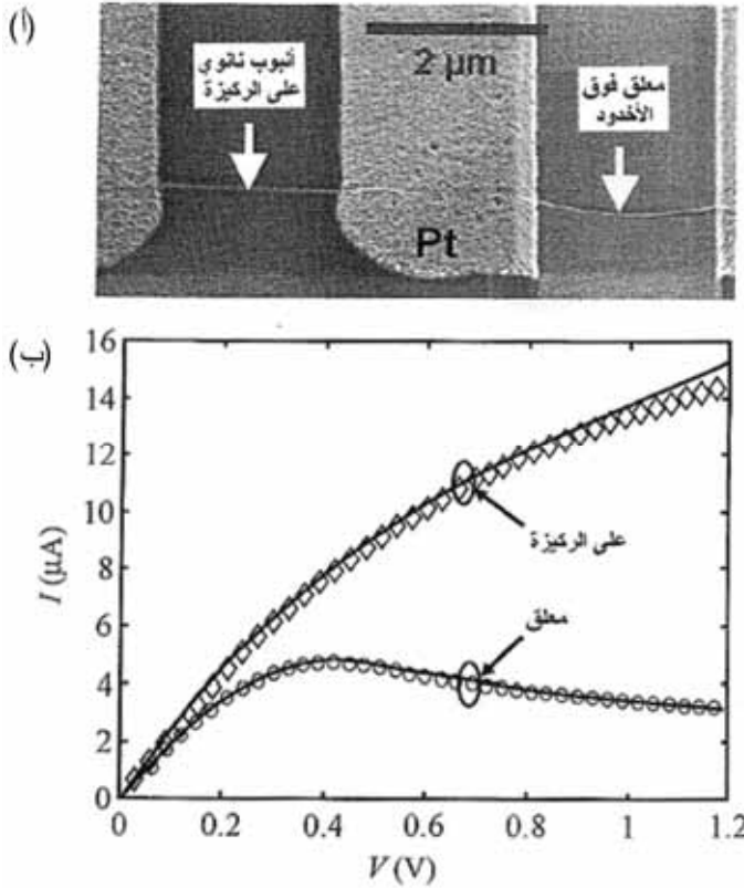
الشكل 11.7: (أ) أنابيب نانوية كربونية على ركيزة ومعلقة على أخدود. (ب) منحنيات التيار بدلالة الجهد
