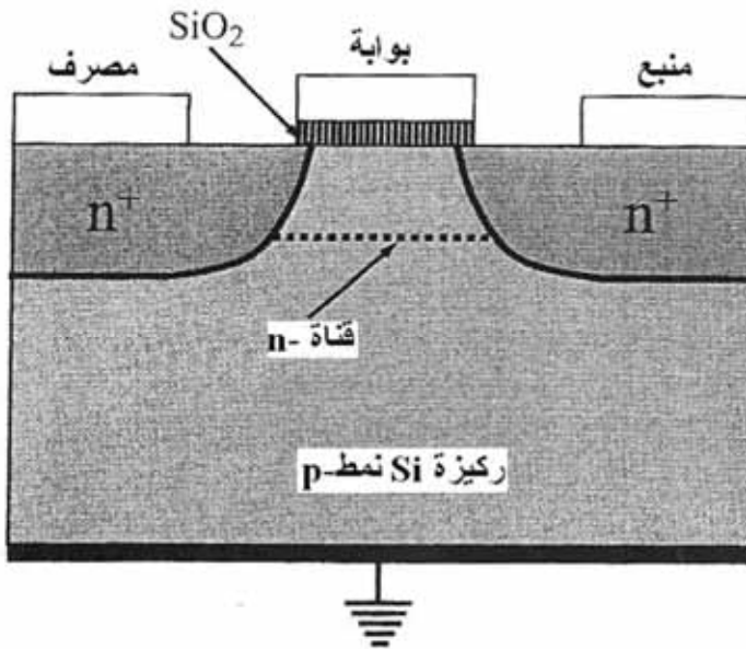
الشكل 12.8: تمثيل لترانزستور MOSFET سيليكوني
