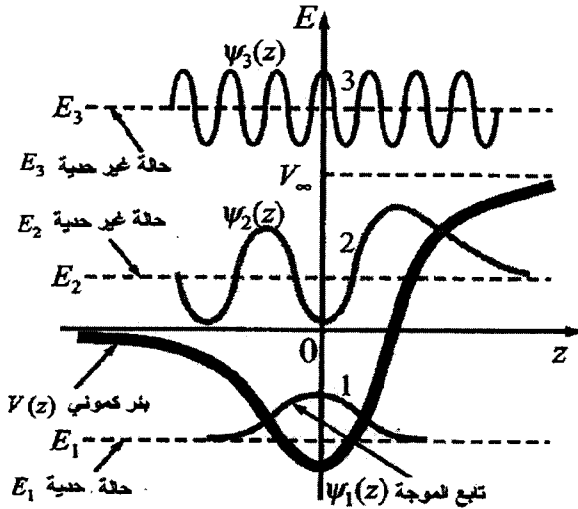
الشكل 1.3: ثلاثة أنواع من حلول معادلة شرودنغر من أجل بئر أحادي البعد ذي شكل اختياري
