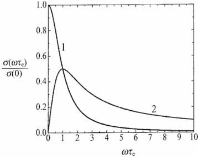
الشكل 9.6: علاقة الجزء الحقيقي (المنحني 1) والعقدي (المنحني 2) لناقلية العنقودية للمعادلة (64.6) بالتردد \omega بالنسبة إلى \sigma(0)=\sigma(\omega=0)
