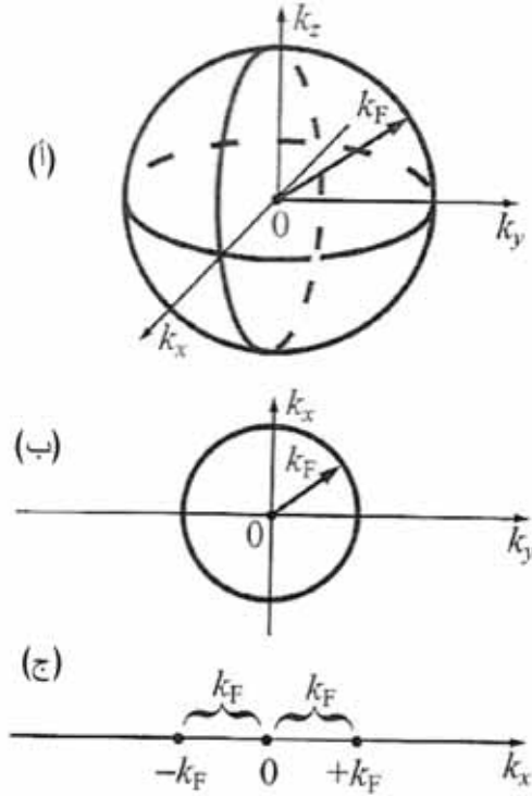
الشكل 5.6: أسطح فيرمي من أجل غاز إلكتروني (أ) ثلاثي الأبعاد و(ب) ثنائي الأبعاد و(ج) أحادي البعد
