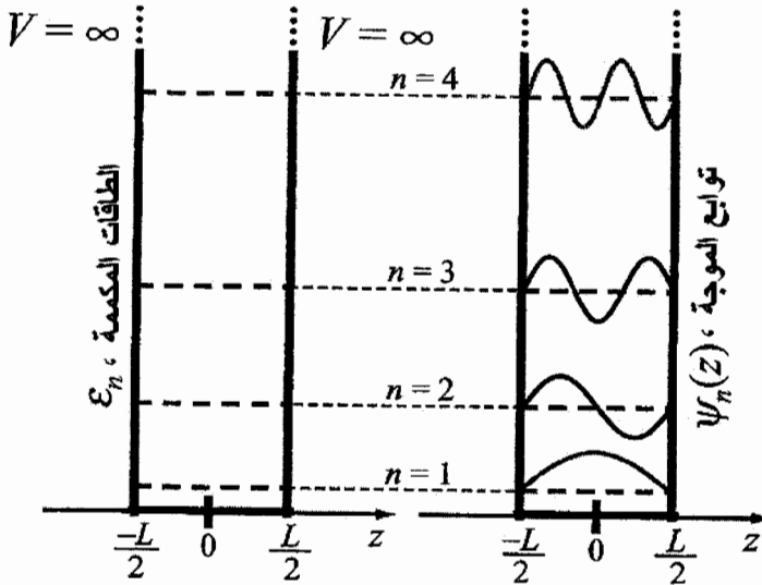
الشكل 2.3: حلول معادلة شرودنجر من أجل بئر كمومي بحدود لانهائية
