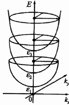
الشكل 7.3: مثال على حزم ثانوية ثنائية البعد. الحزم الثانوية ممثلة بقطع مكافئة في فضاء \{E, k_x, k_y\} النهايات الصغرى للحزم الثانوية \epsilon_1, \epsilon_2, \epsilon_3
