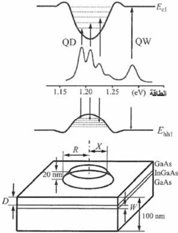
الشكل 13.7: مخطط للكُمونات الحابسة لنقطة كمومية في الإلكترونات والثقوب. توافق قيم الأطياف الضوئية الانتقالات الضوئية بين الحالات المكعبة للإلكترونات والثقوب في النقطة الكمومية
