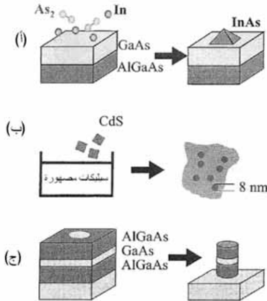
الشكل 12.7: مخطط تمثيلي لثلاث مقاربات لتصنيع النقاط الكمومية: (أ) النمو ذاتي التنظيم لجزر نانوية الحجم. (ب) بلورات نانوية في غراء (ج) نمذجة صناعية وحفر البنية المتباينة مع غاز إلكتروني ثنائي البعد
