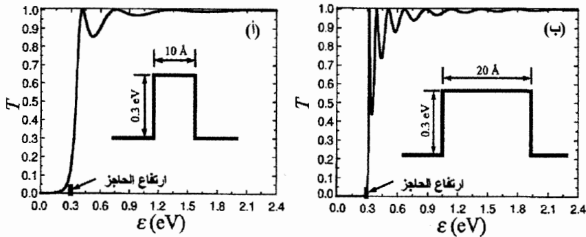
الشكل 14.3: اعتماد معامل الانتقال T على طاقة الإلكترون الوارد \epsilon من أجل عدة سماكات للحاجز L : L=10\text{ \AA} في الحالة (أ) و L=20\text{ \AA} في (ب). ارتفاع الحاجز v_b=0.3e
