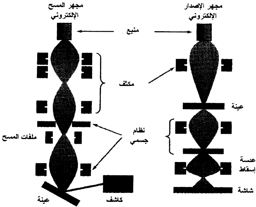
الشكل 12.5: مخطط تمثيلي لمجهر المسح الإلكتروني SEM ومجهر الإصدار الإلكتروني
