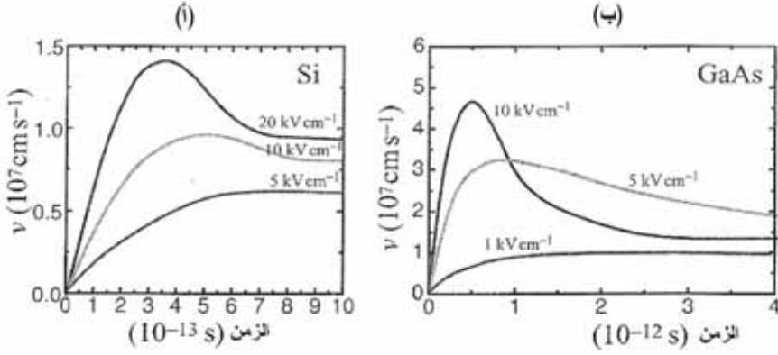
الشكل 13.6: أثر التجاوز - الاستجابة العابرة لسرعة انزياح الإلكترون بسبب نبضات حقل كهربائي شبيهة بتابع الدرجة في درجة حرارة الغرفة. قيمة الحقل المذكورة من أجل كل منحني. (أ) Si و (ب) GaAs
