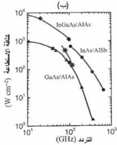
الشكل 8.8: (أ) الدارة الكهربائية الأيسر. (ب) طاقة الأمواج الميكروية المولدة في وحدة سطوح مقطع الديودات النفقية التجاوبية الثنائية الحاجز كتابع للتردد لنفس أدوات الشكل 7.8 (ب)
