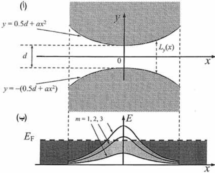
الشكل 18.6: تمثيل هندسي لنقطة الوصل (أ) والطاقة المكممة E_{1,m} في منطقة نقطة الوصل (ب). يظهر أن الإلكترونات يمكن أن تكون في كل الحزم الجزئية في المنطقة الغامقة. أما في المنطقة الفاتحة فيمكن أن تكون الإلكترونات في الحزمة الجزئية \varepsilon_{1,1}
