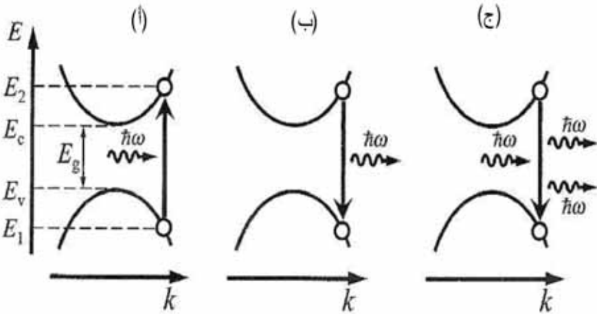
الشكل 43.8: (أ) يعطي امتصاص الفوتون تحريض زوج إلكترون-ثقب. (ب) إصدار تلقائي يمكن تفسيره بإعادة ارتباط إلكترون-ثقب. (ج) إصدار محفز
