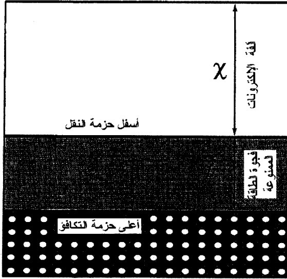
الشكل 11.4: يمثل هذا المخطط ألفة الإلكترون ومستوى الفراغ في بلور
