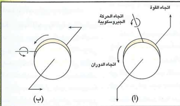
● شكل (14)، اتجاه الحركة الجيروسكوبية.
