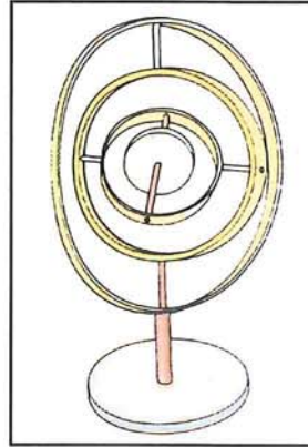
● شكل (٦)، جيروسكوب فثائي درجة الحرية.
