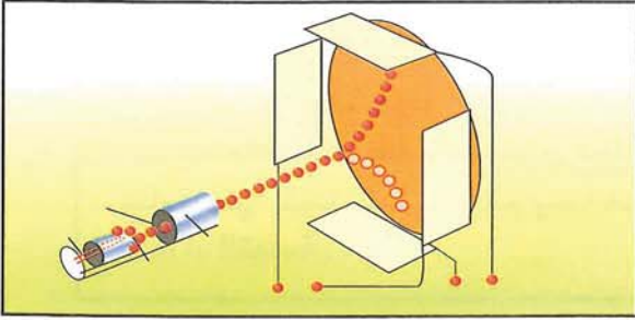
● شكل (2) مكونات صمام الأشعة المهبطية.
