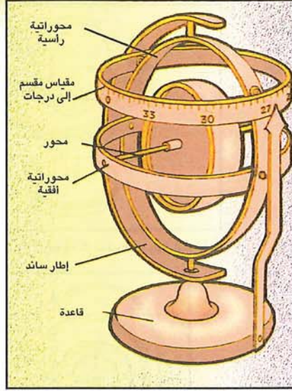
● شكل (3)، جيروسكوب الطائرات.
