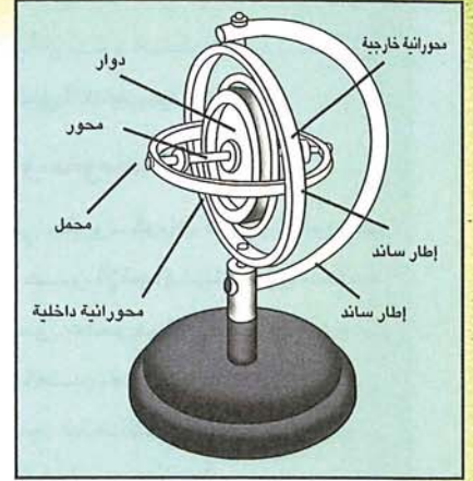
● شكل (2)، الأجزاء الرئيسية للجيروسكوب.
