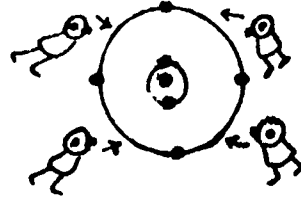
اربعة ذرات ايدروجين تحيط بذرة من الكربون
