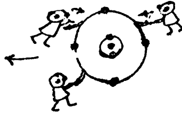
في الوسط ذرة من النيتروجين تبيع لها شريعتها الأليكترونية الارتباط بثلاث ذرات من الأيدروجين
