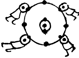
وعندما تتزوج الكربون بالاربعة يصبح على هيئة جزىء غاز المستنقعات
