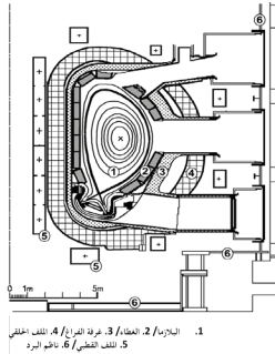
رسم توضيحيّ ٩. رسم قطاعي للمفاعل النووي الحراريّ التجريبيّ الدوليّ
