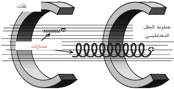
رسم توضيحي ٤. مسار أيون (+) وإلكترون (-) في حقل مغناطيسي ثابت
